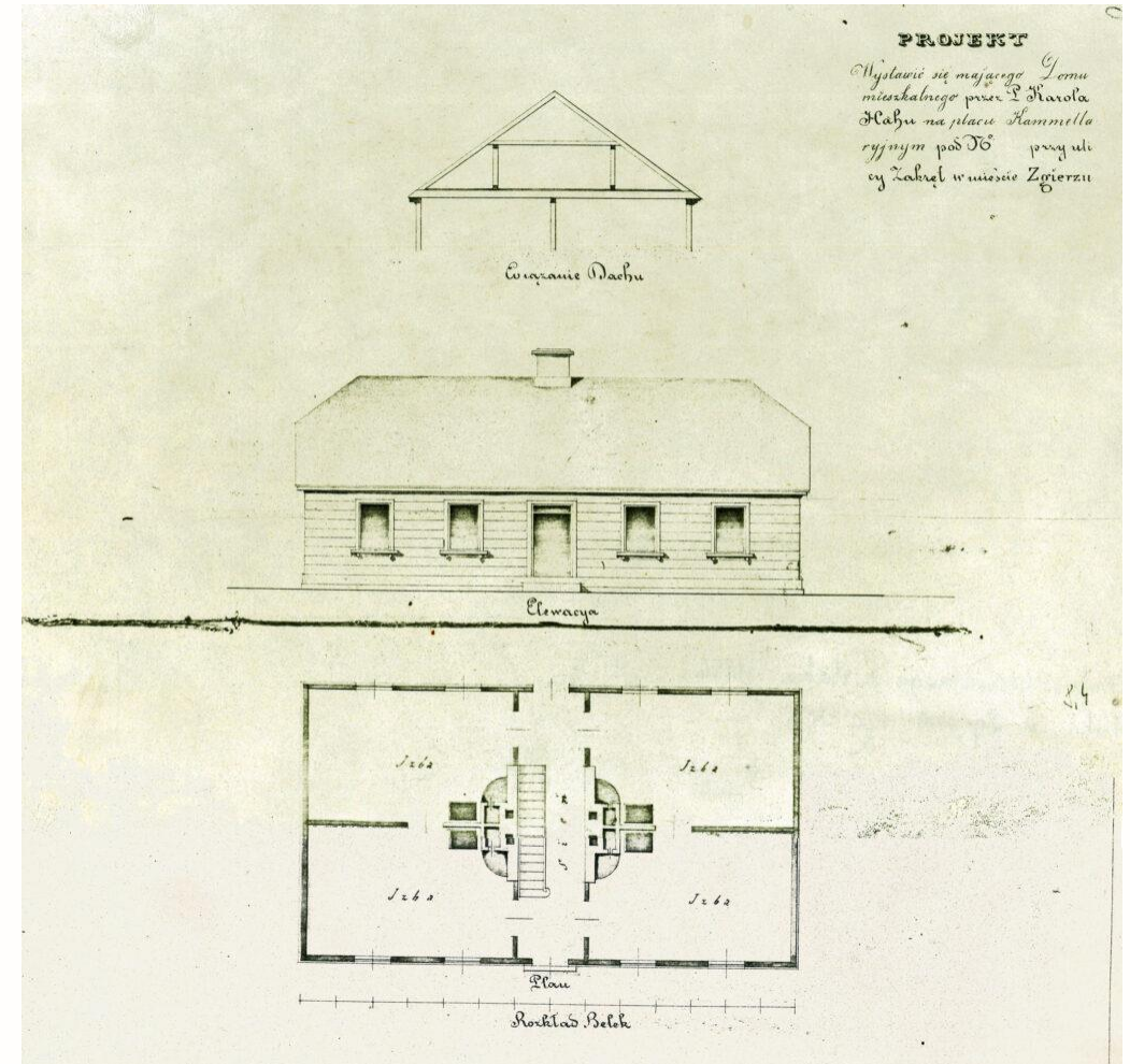
Projekt domu tkacza z ulicy Zakręt w Zgierzu (Archiwum Państwowe w Łodzi)
